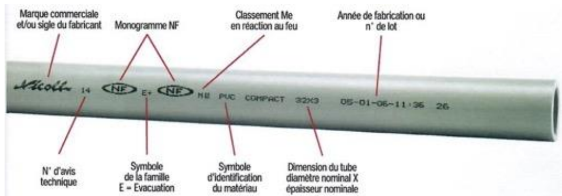
Image 1 : Codification des tuyaux
