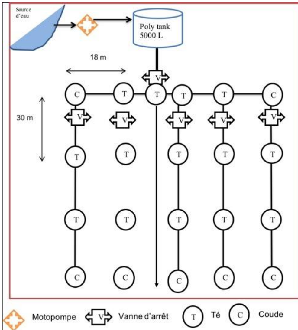
Figure 8 : Plan de répartition des composants du réseau
